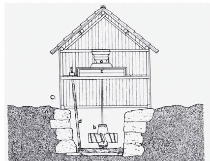
Figur 55 Skvaltkvarn i genomskärning. Såden matas in i den trattliknande anordningen (a) Själva skvaltän hade en vertikal axel (b), och drev den rörliga kvarnstenen (c) direkt. Genom att dra bjälken (d) uppåt kunde man lyfta upp axeln för justering av luftspalten mellan kvarnstenarna.
