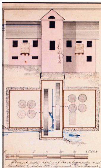
Ritning på kvarnen från kartan daterad 1851. I mitten ser man de två stora vattenhjulen som på var sin horisontella axel via en enkel kuggväxel driver vardera fyra par kvarnstenar. De blå strecken visar troligen vattenledningen/rännan och nere till höger ser man hur vattnet rinner ut.
